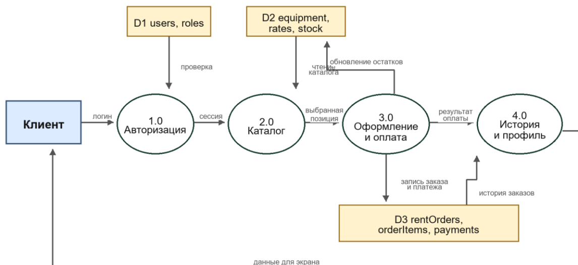
Рис. 5. Диаграмма потоков данных DFD уровня 0
