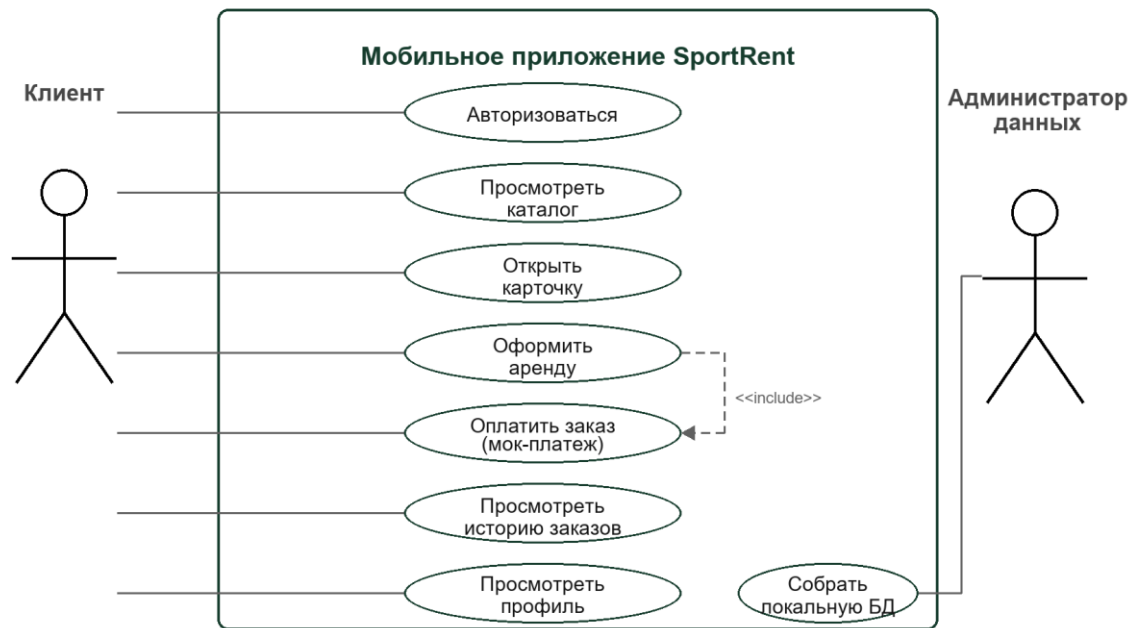
Рис. 2. Диаграмма вариантов использования SportRent
